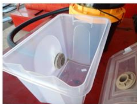
Figura 11.2 – Detalhe da tela de retenção na caixa de captura (Fonte: Comissão)
